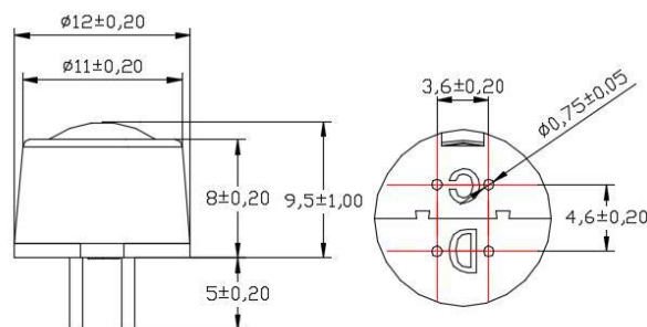
图 1： 传感器外形结构
