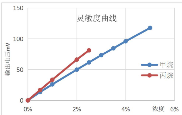
图 3：灵敏度曲线
