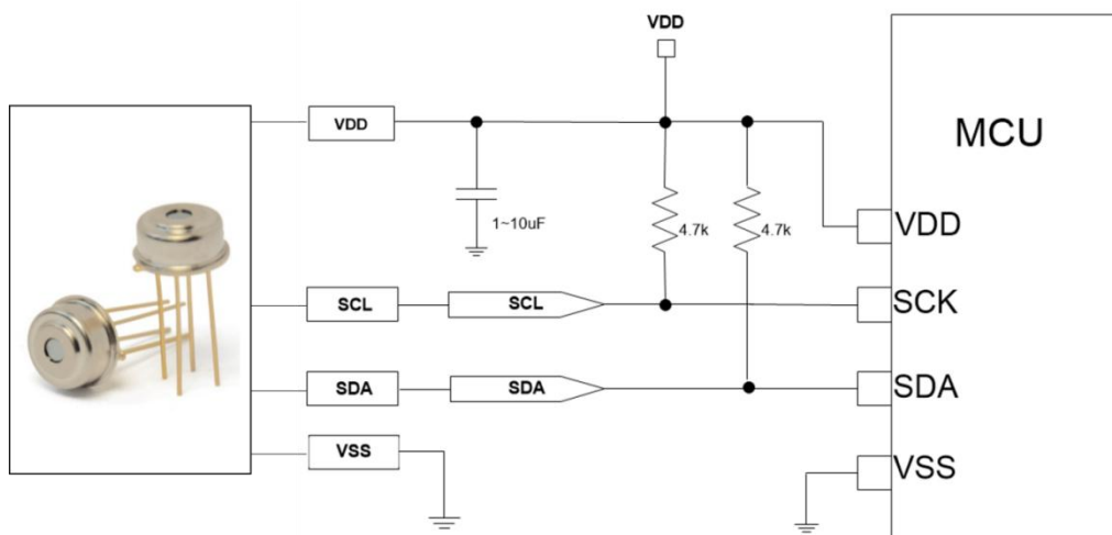
图 9: 推荐电路
