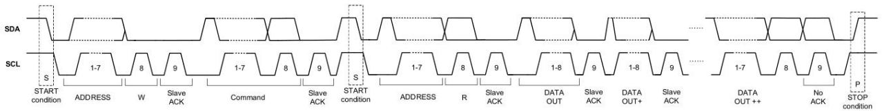
图 7: I 2 C 正常模式 I 2 C 分组读取
