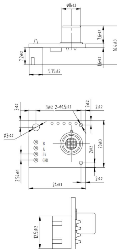
图 1: 模组结构图
