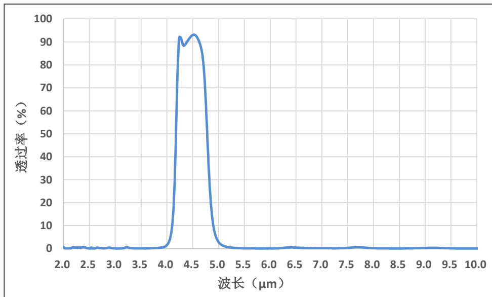
4. 48µm 窄带滤光片光谱曲线
