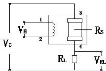
图 2：MP-2 测试电路
