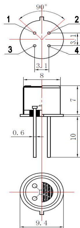
图 1 元件外形结构
