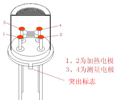
图 7： 管脚示意图
