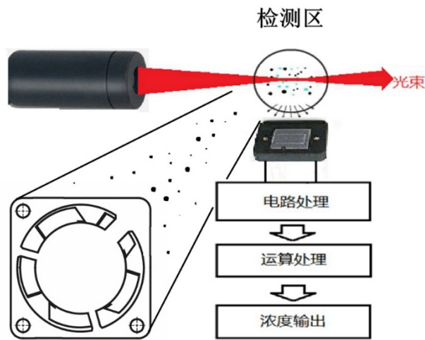
图3-原理说明
