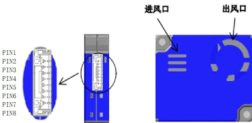
图 1-引脚顺序
